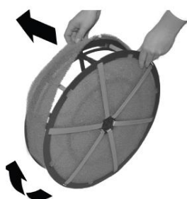
Рис. 22 Удаление внешнего барабана фильтра испарителя
