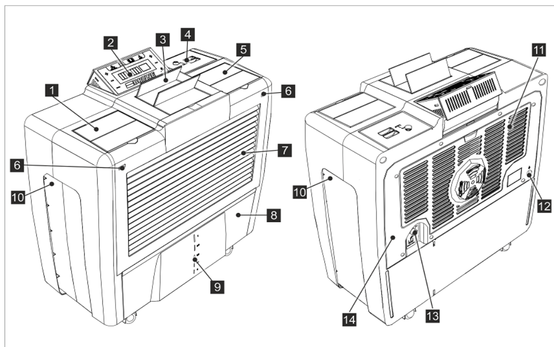
рис. 1 — Общий вид увлажнителя
